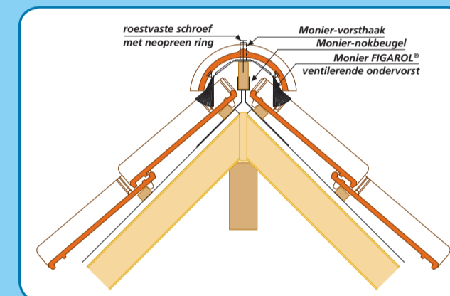
Nokdetail halfronde vorst
