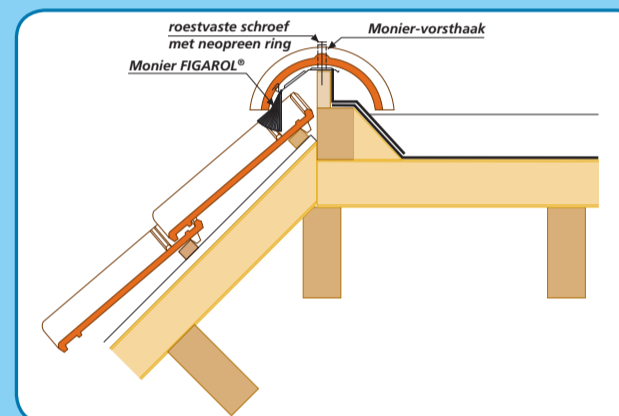
Aansluiting nok met plat dak
